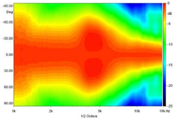
Horizontal Beamwidth
